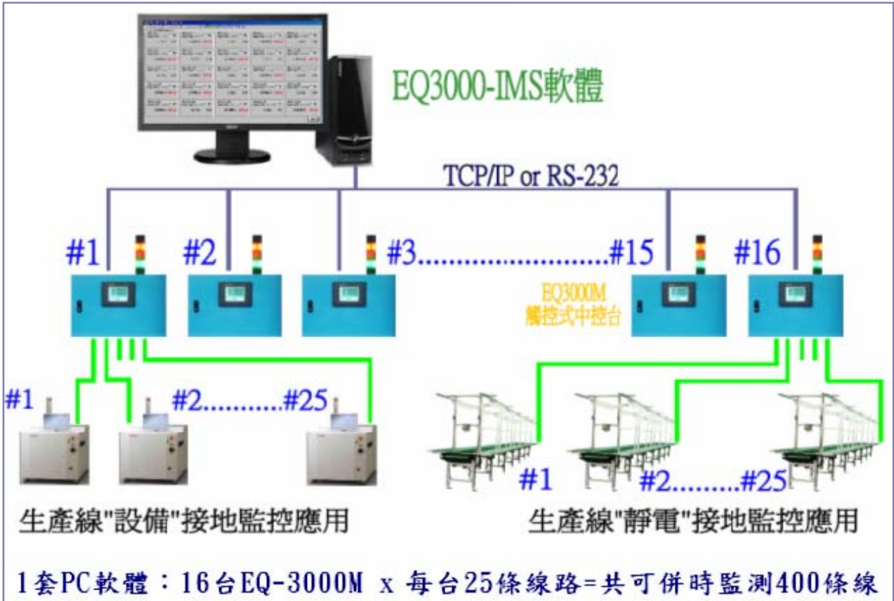
EQ-3000-IMS 中控管理之系統整體監控示意圖
