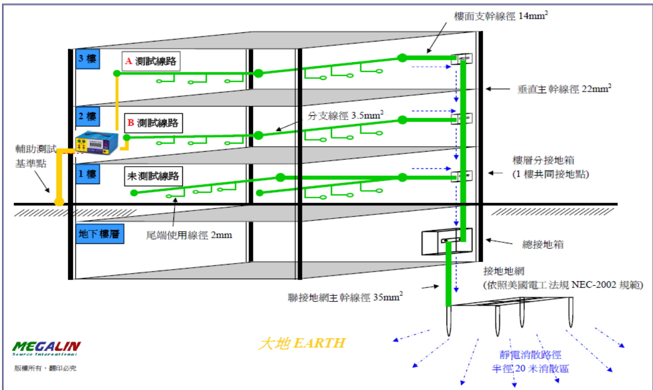
EQ-3000/EQ-3000M 交流阻抗監測器使用示意圖
